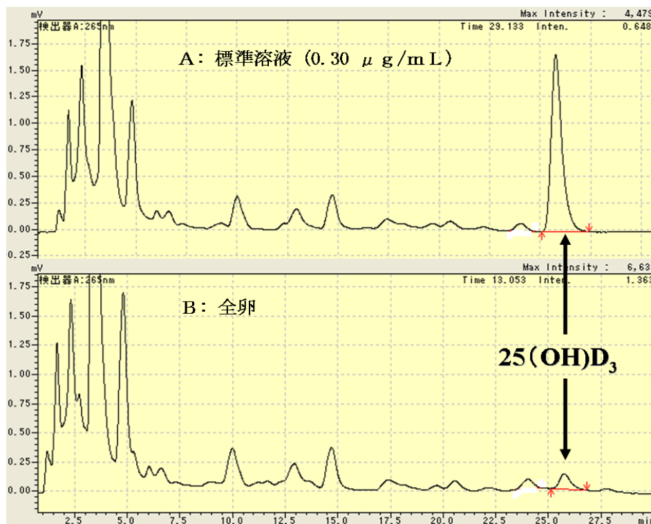
図-2 標準溶液(A)と全卵(B)のクロマトグラム
